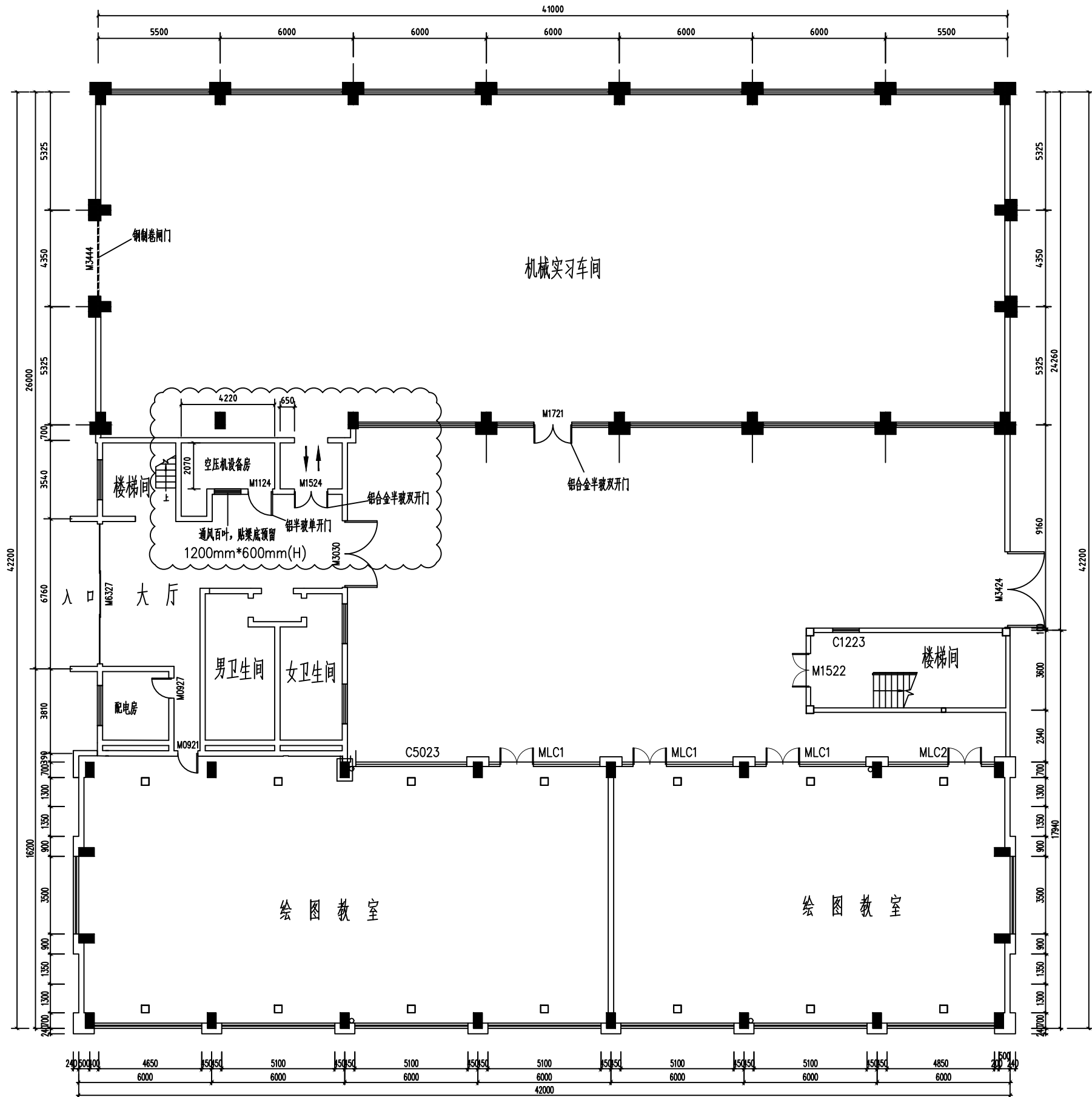
制图楼+ 机械实习车间一层平面 1 : 1 0 0
