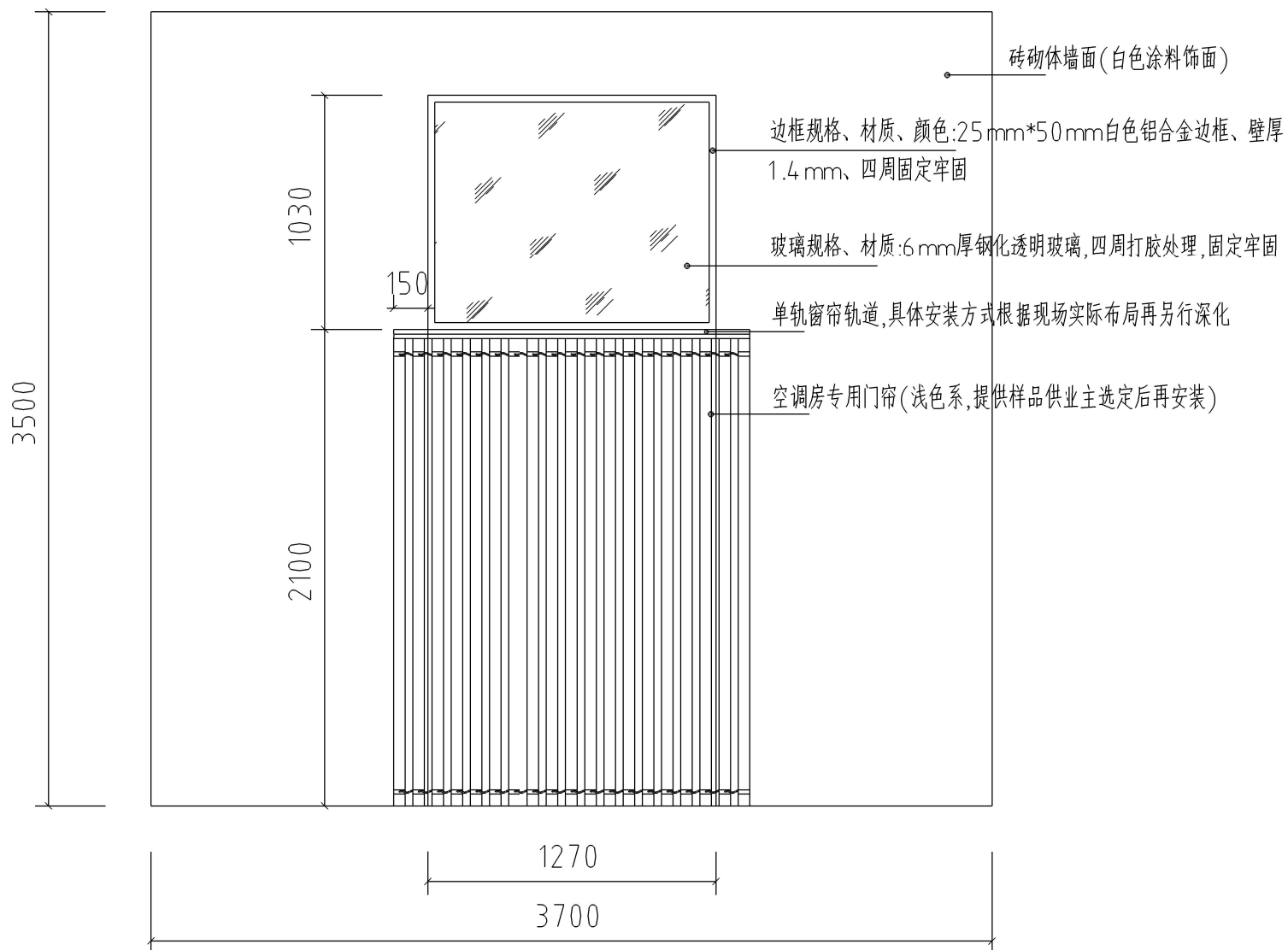
成园宿舍房间隔断示意图
